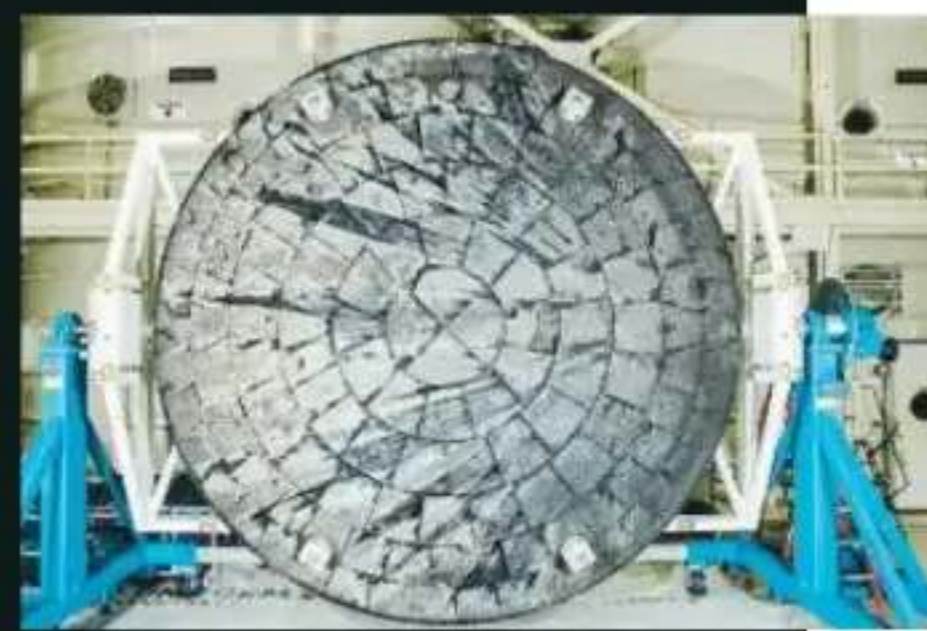
El escudo térmico de la Orión de Artemis I después del amerizaje
